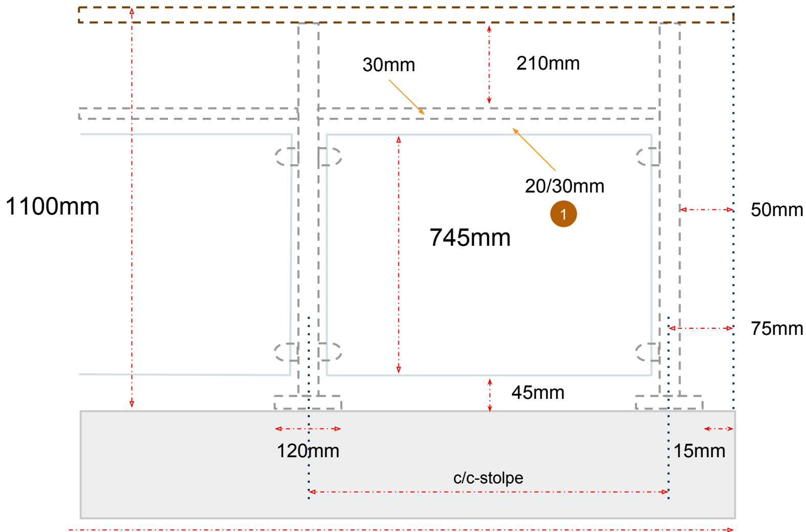
Måttagning, kant till kant
